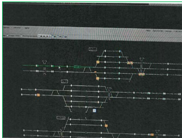
Vedere CIM – RBC - trenul 17153 circulă în ECTS nivel 2
