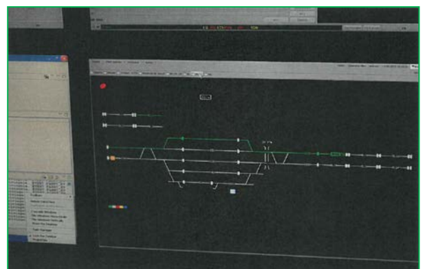
Vedere CIM – RBC – autorizația de mișcare pentru trenul 17153 este în concordanță cu parcursul comandat în Stația Periș
