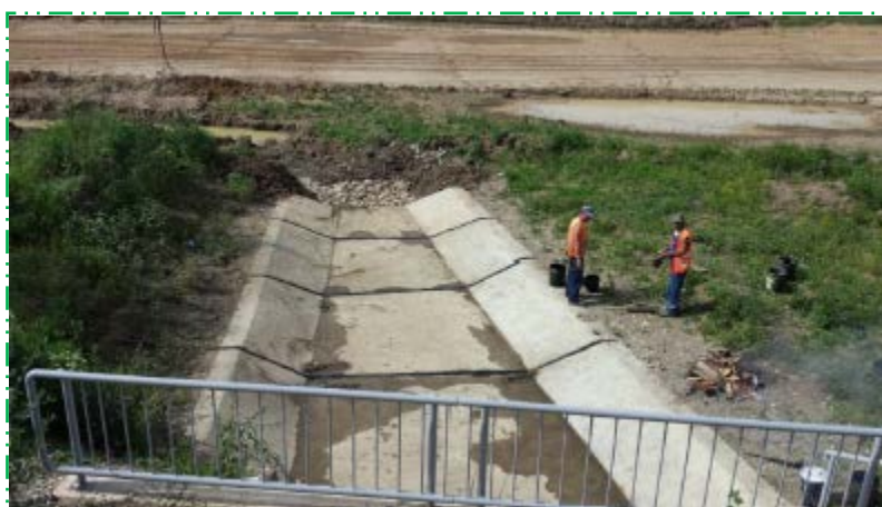
Realizare saltea piatră brută albie aval
