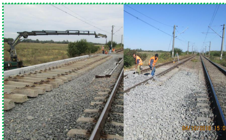
Montare traverse S.B. și completare prismă piatră spartă – Fir I
