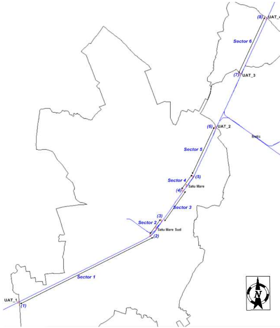
Figura nr 1 Delimitarea sectoarelor de cale ferată considerate în cadrul Unității Administrativ Teritoriale
