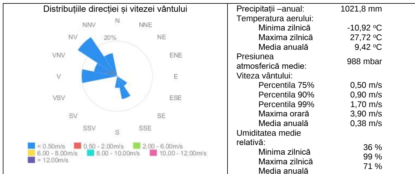
Fig. nr. 1: Valorile parametrilor meteorologici înregistrați în anul 2021 în municipiul Baia Mare) (Latitudine: 47.6517258 Longitudine: 23.5705070 Altitudine: 223.00 m) (sursa: CalitateAer - Rețeaua Națională de Monitorizare a Calității Aerului www.calitateaer.ro )
