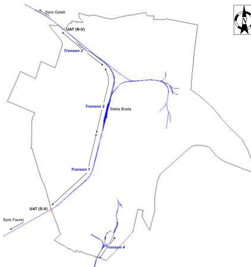
Fig. nr. 2: Delimitarea segmentelor de cale ferată în cadrul Aglomerării – sursa CNCF CFR SA
