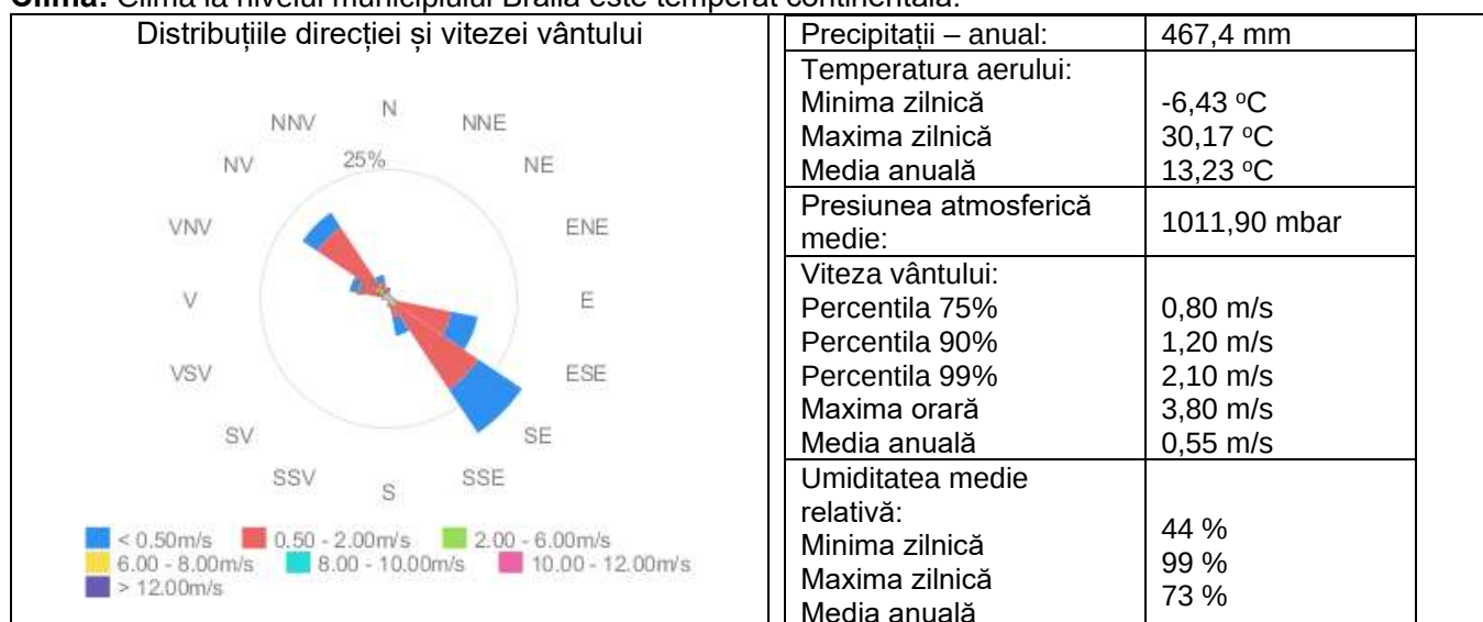
Fig. nr. 1: Valorile parametrilor meteorologici înregistrați în anul 2021 în municipiul Brăila)
