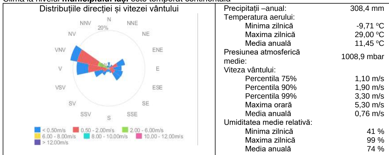
Fig. nr. 1 Valorile parametrilor meteorologici înregistrați în anul 2021 în municipiul Iași) (Latitudine: 47.1509514 Longitudine: 27.5819187 Altitudine: 42.00 m) (sursa: CalitateAer - Rețeaua Națională de Monitorizare a Calității Aerului www.calitateaer.ro )
