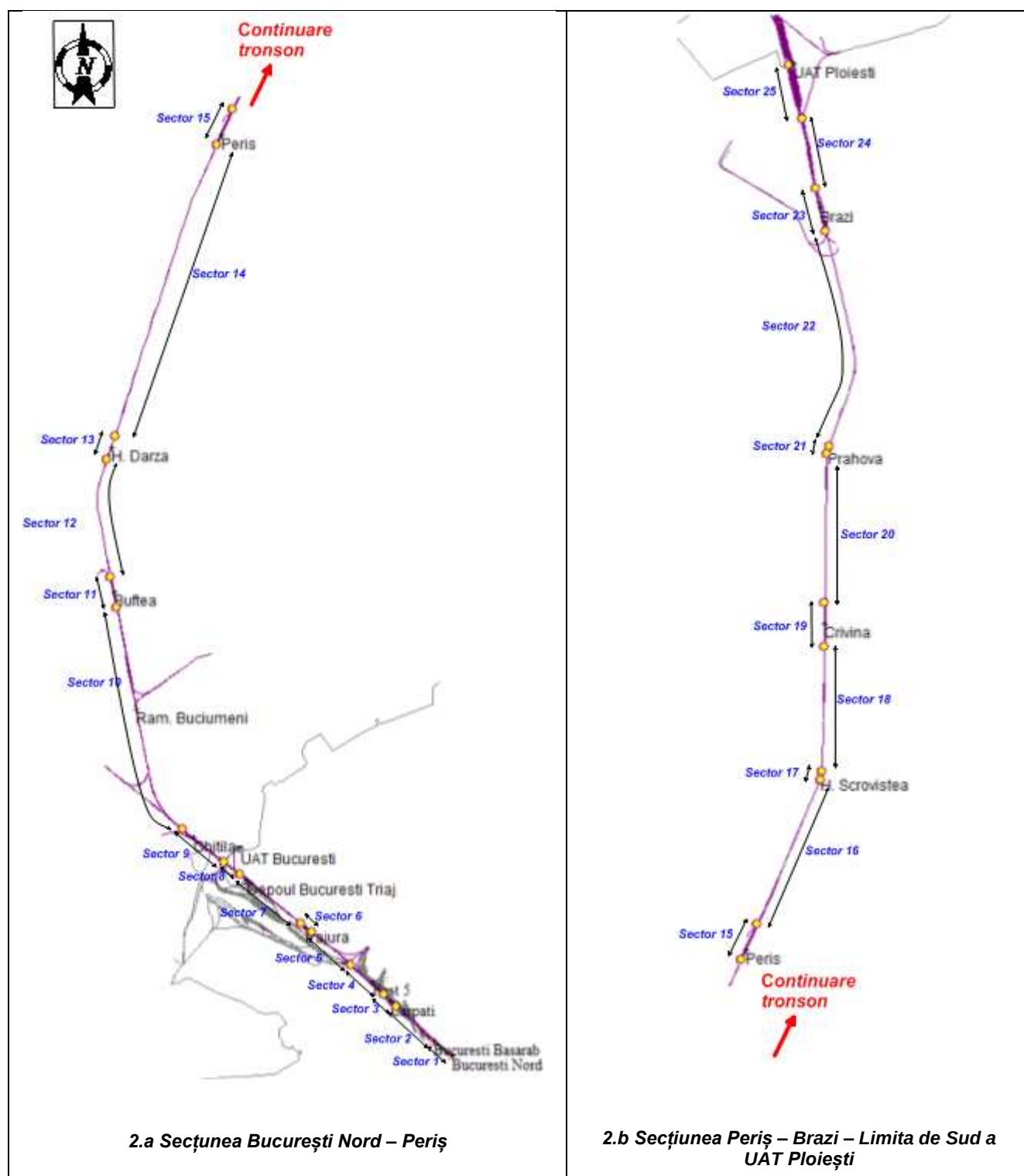
Figura nr 2 Delimitarea segmentelor de cale ferată principală considerate de-a lungul tronsonului București – Brazi – Limita de Sud a UAT Ploiești
