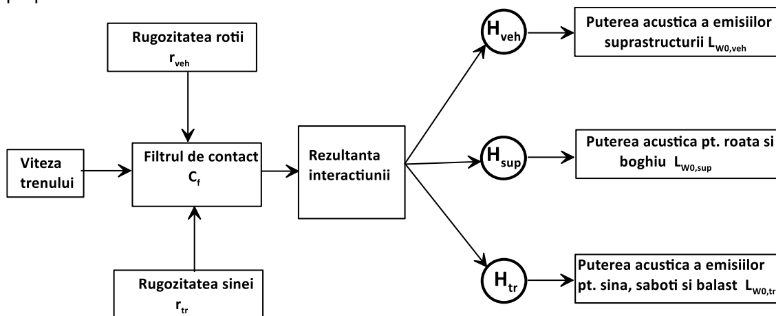
Fig. nr. 5 Reprezentarea mecanismului de generare a zgomotului (parametrul putere acoustică), urmare a interacțiunii roată – șină. Unde:
