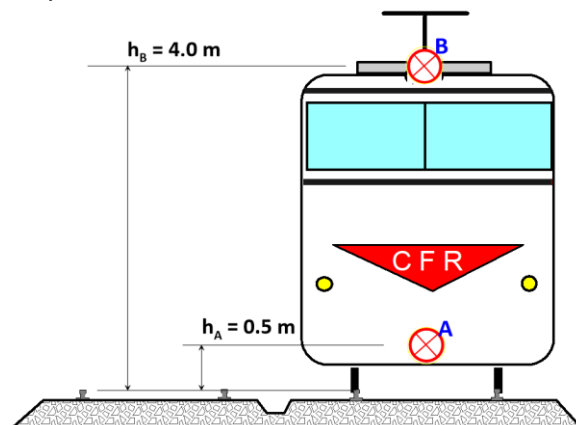
Fig. nr. 2 Amplasarea surselor de zgomot echivalente
