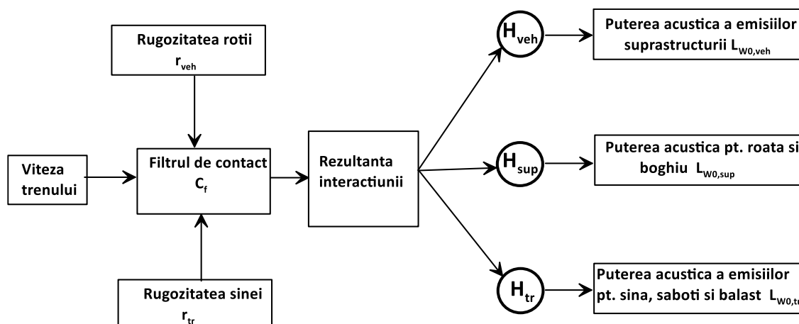
Fig. nr. 4 Reprezentarea mecanismului de generare a zgomotului (parametrul putere acustică), urmărirea interacțiunii roată – șină. Unde:
